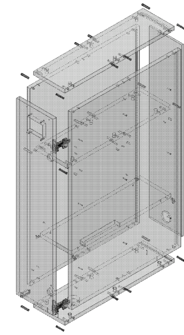
Explosionszeichnung
