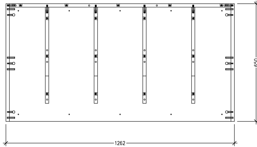
Draufsicht
