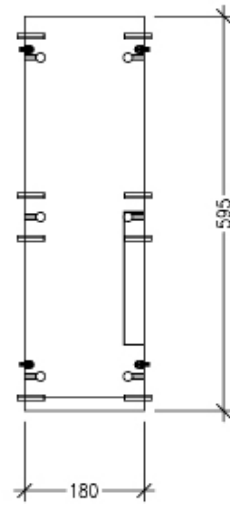
Draufsicht
