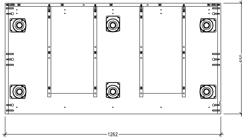
Draufsicht
