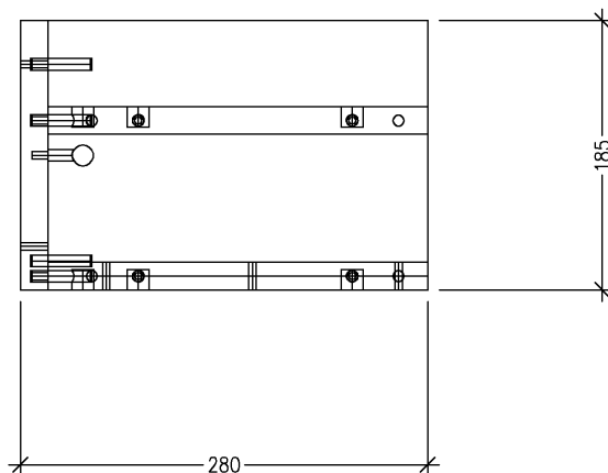
Frontansicht
