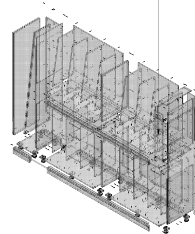
Explosionszeichnung
