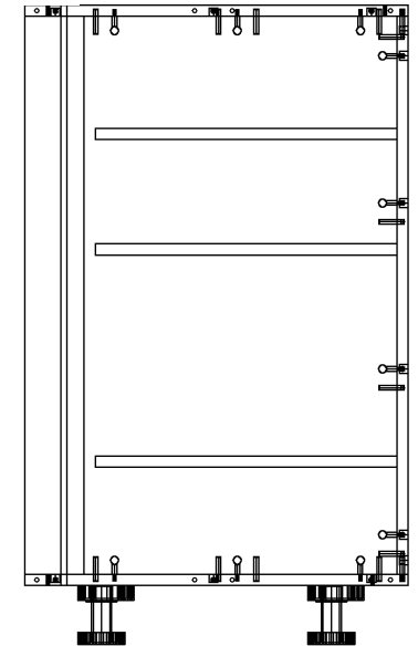
Seitenansicht rechts
