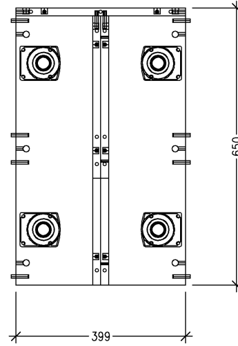
Draufsicht
