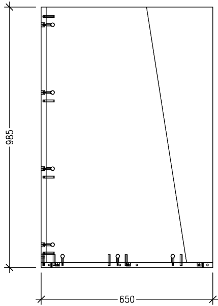
Seitenansicht links
