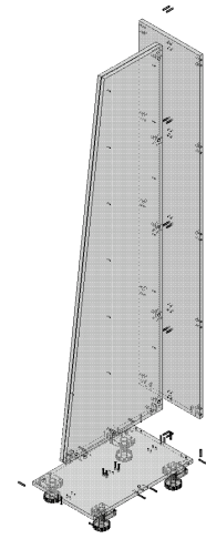
Explosionszeichnung
