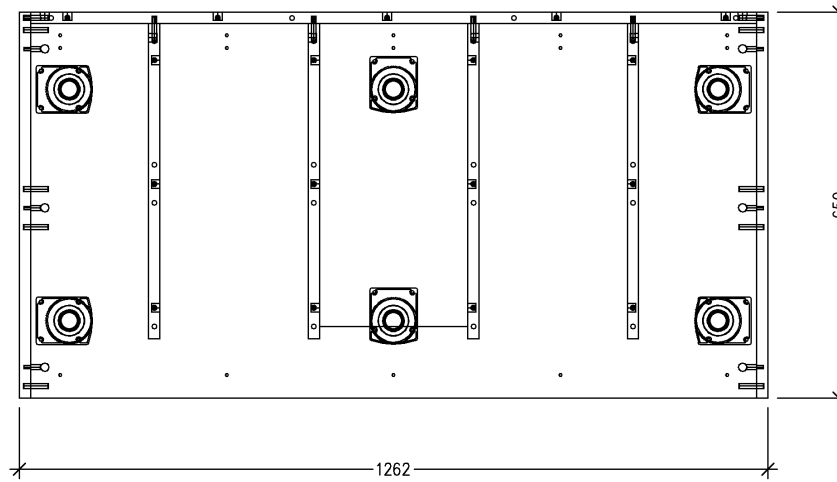
Draufsicht
