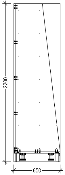
Seitenansicht links
