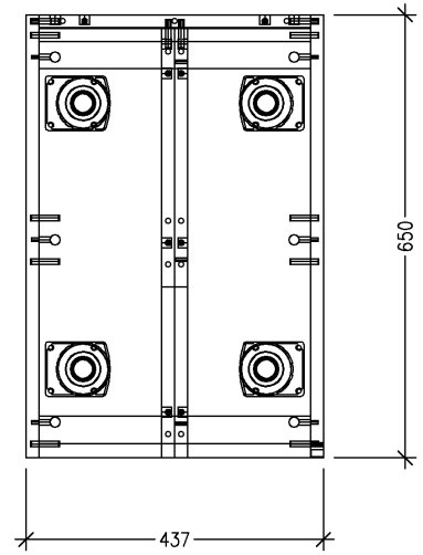
Draufsicht
