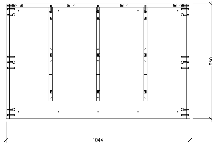
Draufsicht
