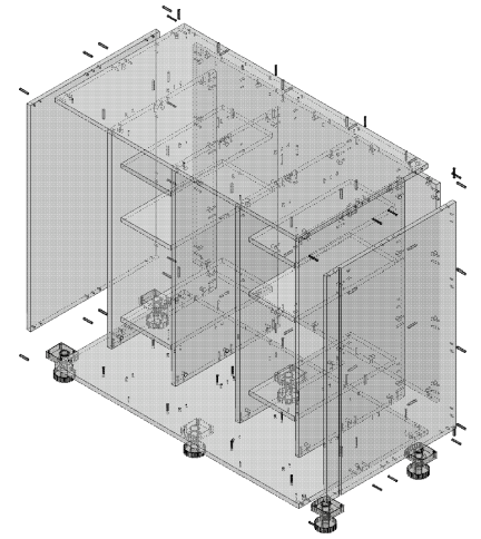
Explosionszeichnung
