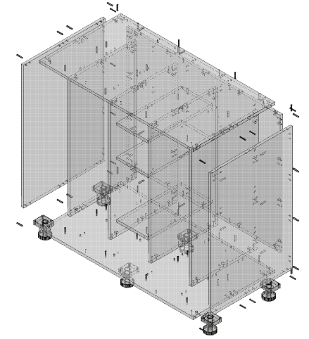
Explosionszeichnung
