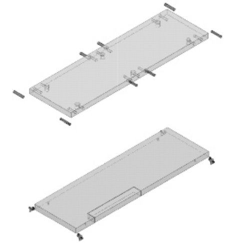
Explosionszeichnung
