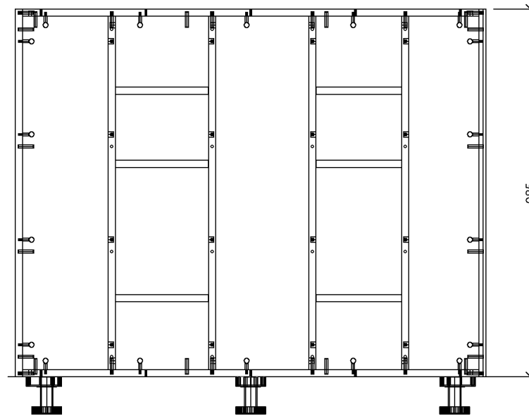
Frontansicht
