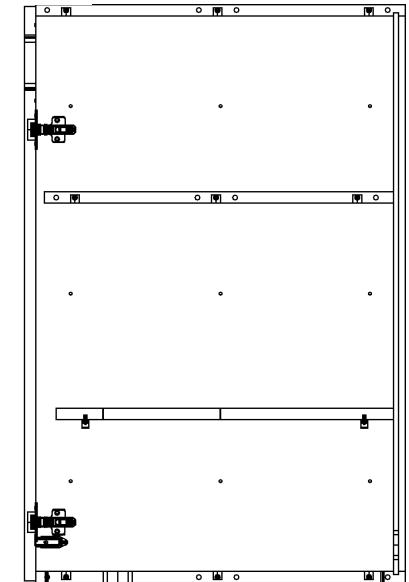
Seitenansicht rechts
