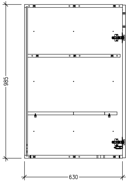
Seitenansicht links
