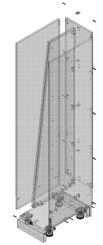
Explosionszeichnung
