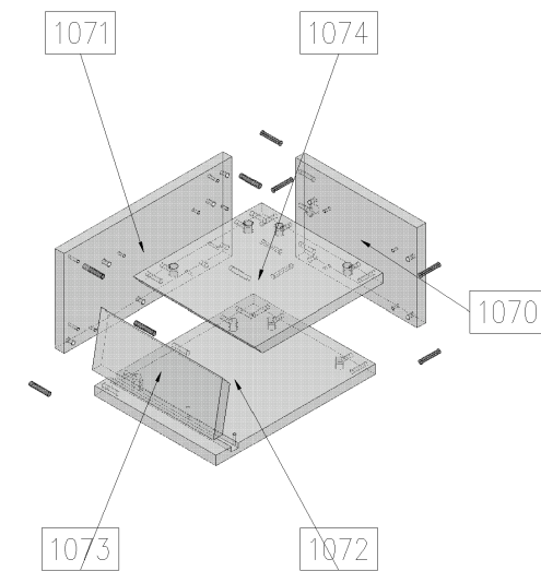
Explosionszeichnung
