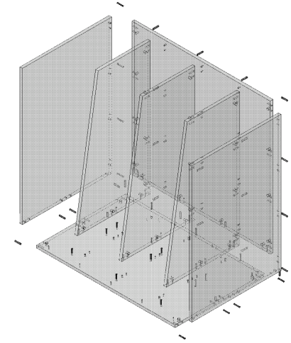
Explosionszeichnung
