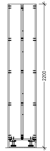
Frontansicht
